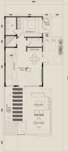
الدور الثاني:
