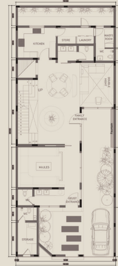
الدور الأرضي:
